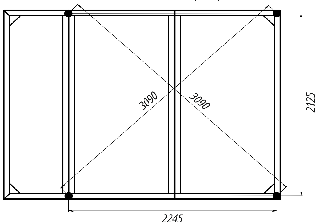
Схема разметки свайного поля для бани размерами 2300х3100
