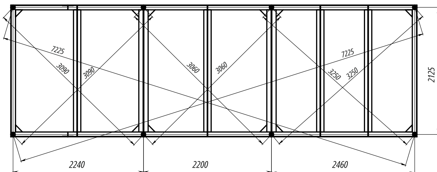
Схема разметки свайного поля для бани размерами 2400×7150
